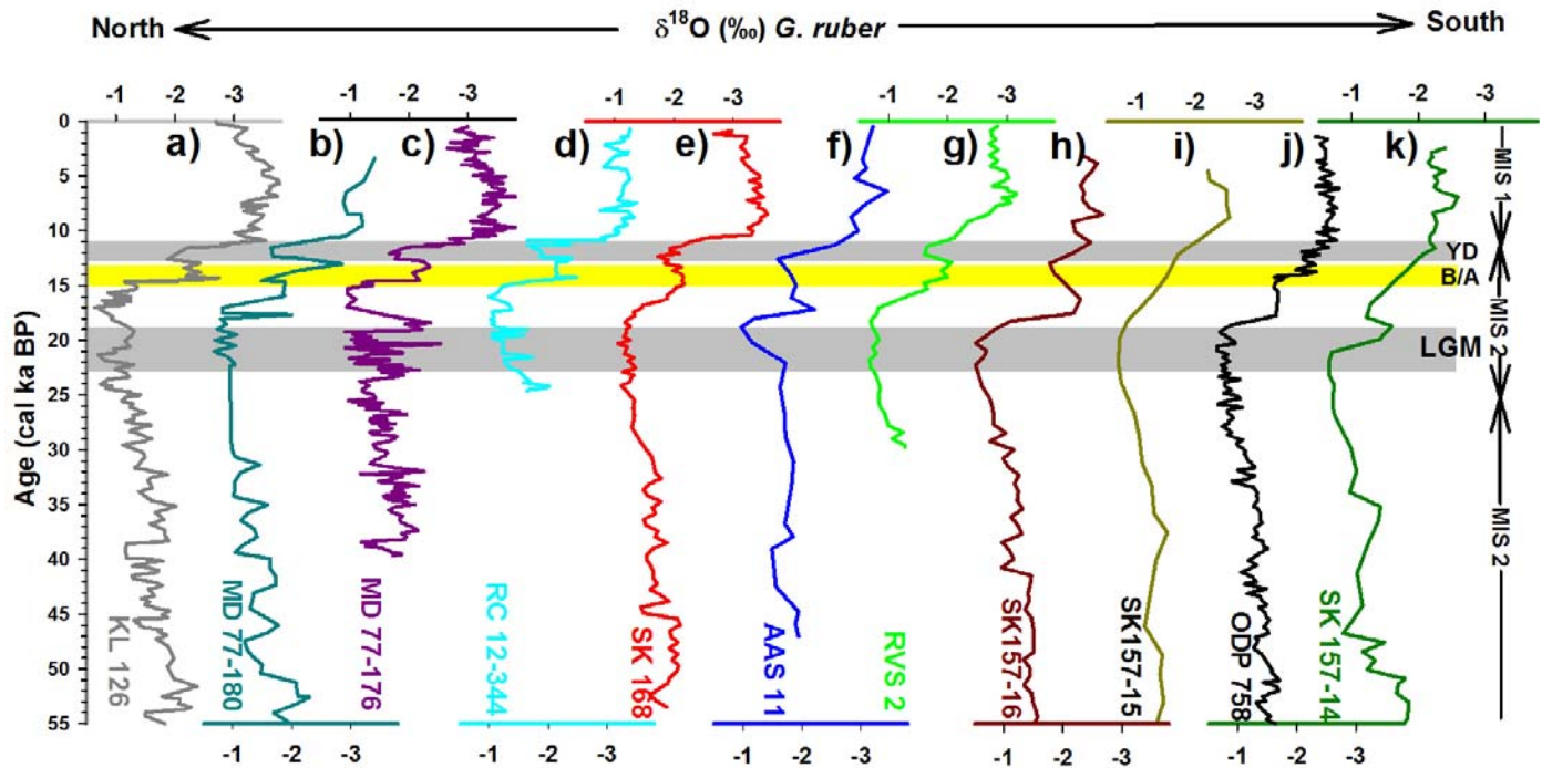
Fig. 6. G. ruber (mixed layer) oxygen isotope records a) core KL 126 (Kudrass et al., 2001); b) core MD 77-180 (Duplessy, 1996; Colin et al., 1998); c) MD77-176 (Marzin et al., 2013); d) RC 12-344 (Rashid et al., 2007); e) SK 168 (Sijinkumar et al., 2010) f) AAS 11 (Ahmad et al., 2000); g) RVS 2 (Sijinkumar et al., 2015) h) SK157-16 (Raza et al., 2014); i) SK 157-15 (Raza et al., 2014); j) ODP 758 (Bolton et al., 2013); k) SK 157-14 (Ahmad et al., 2008).
