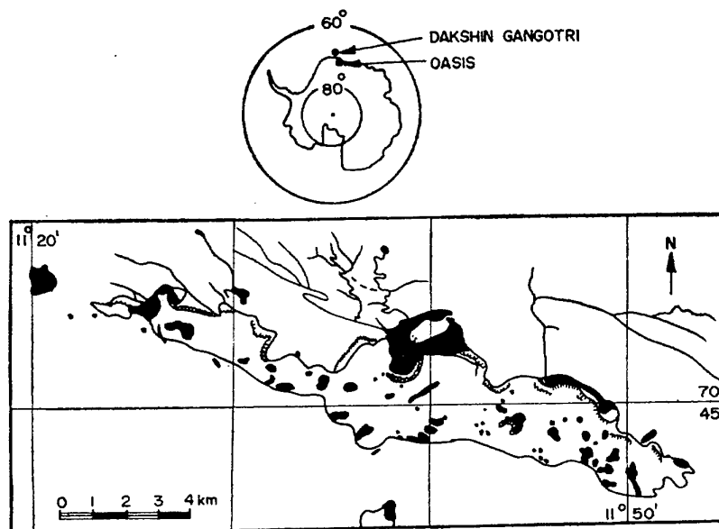
Fig. 1. Schirmacher Oasis, Antarctica
