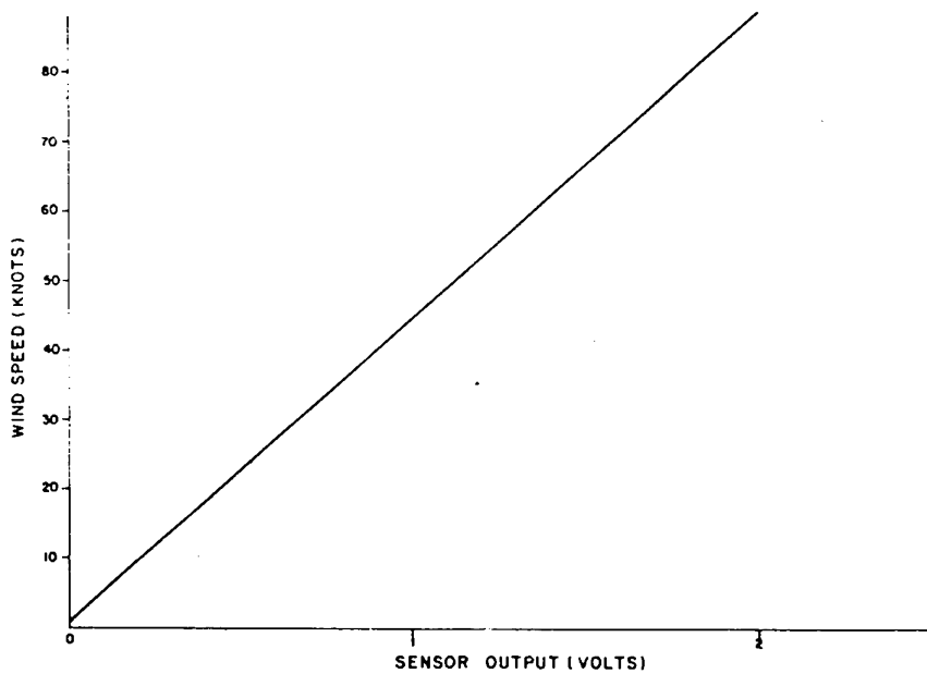
Fig. 2 : Cup anemometer calibration chart.
